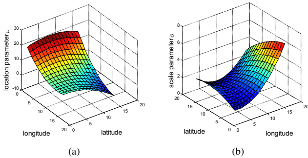
Fig. 3. True GEV parameters for synthetic data: (a) Location parameter surface; (b) Scale parameter surface.
